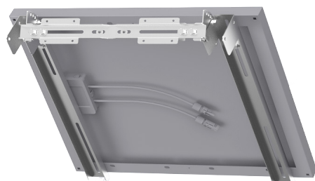
UNIFIX 50 Pour Unisun 30.12M/ 50.12M/ 50.24M/ 55.12BC Orientation paysage Ref 0279
