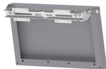
UNIFIX 20 Pour Unisun 10.12M/ 10.24M/ 20.12M/ 20.24M Orientation paysage Ref 0262
