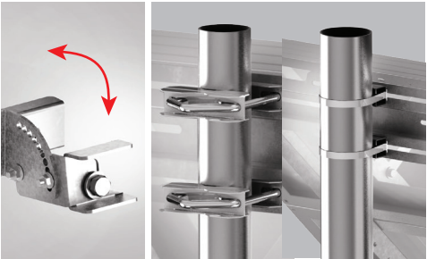
Système d'inclinaison multi-position pour optimiser vos performances électriques Serrage robuste et puissant sur mâts ronds grâce aux brides incluses Se fixe sur tous les supports de signalisation (brides à prévoir)
